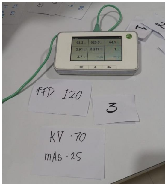
Gambar 4. Hasil Pengujian Output Radiasi (Sumber: Astari, 2026)
